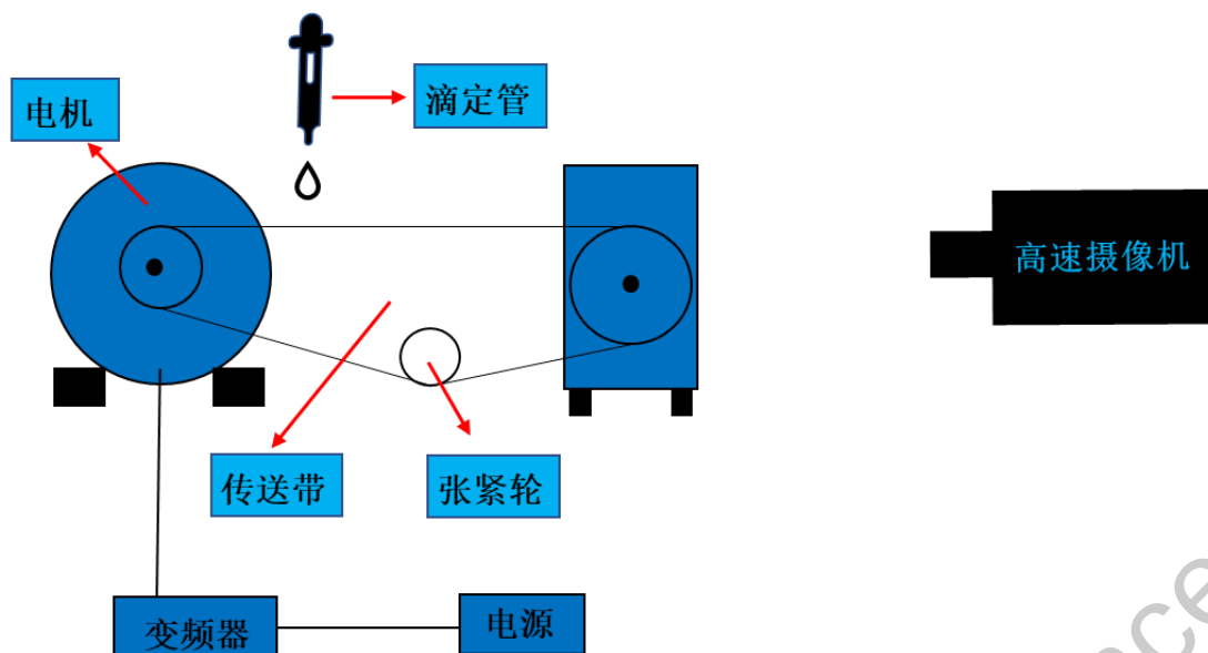
图 16 实验装置模拟图
