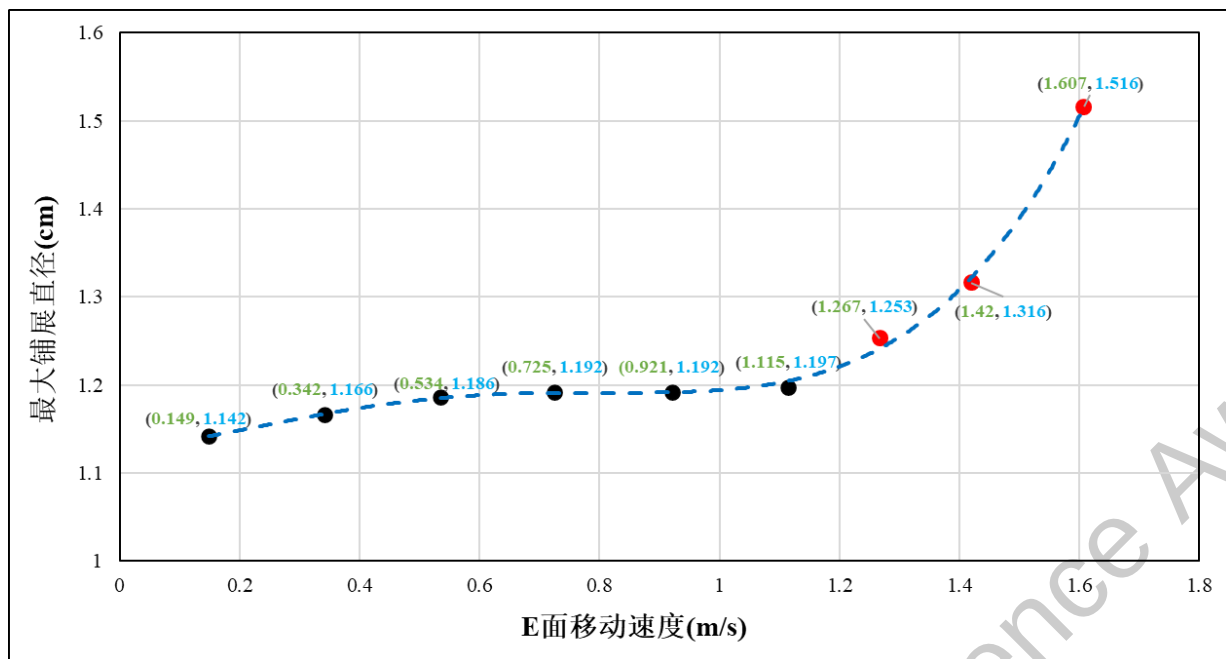
图 21 液滴最大铺展直径与 E 面运动速度间的关系
